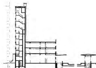
CORTE C-C TORRE - EDIFICIO CENTRAL - PASEO - SALA INTEL. - AREA DE OLA
