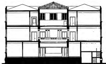
CORTE
