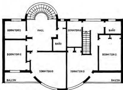
PLANTA 2º NIVEL
