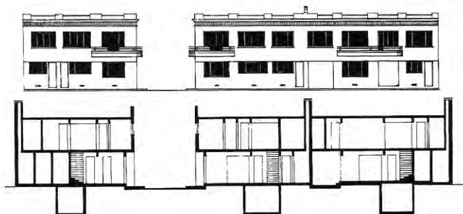
CORTE W-W
