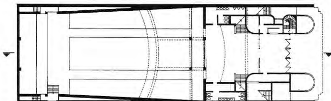
PLANTA PRIMER NIVEL
