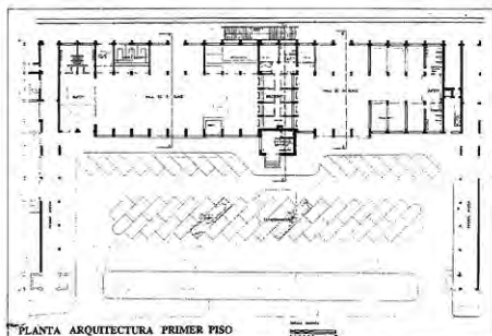
PLANTA ARQUITECTURA PRIMER PISO
