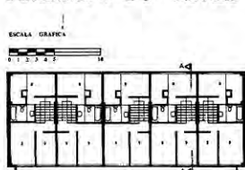
PLANTA 6º Y 7º NIVEL
