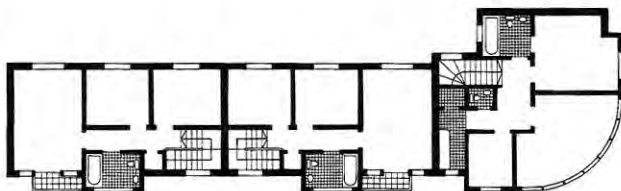
PLANTA PRIMER NIVEL
