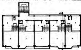
PLANTA 4º Y 5º NIVEL
