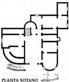
PLANTA SOTANO
