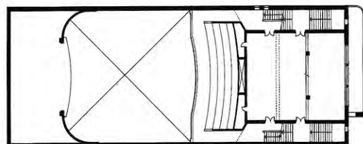
PLANTA 2º NIVEL
