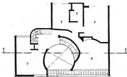
PLANTA 2º PISO
