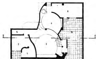
PLANTA 1º PISO
