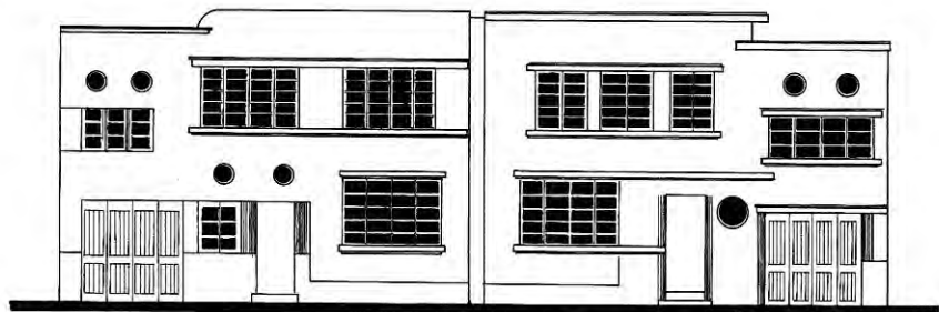
ELEVACION CALLE MAIPU
