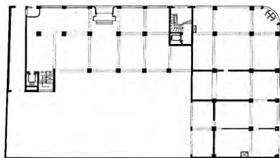
PLANTA 1° PISO
