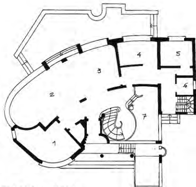
PLANTA 1 er PISO
