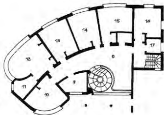
PLANTA 2 o PISO
