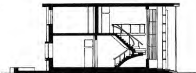
CORTE
