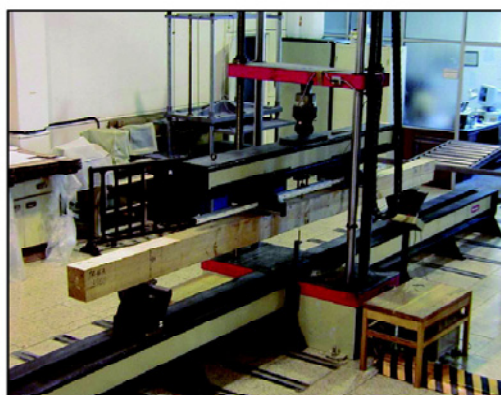
Figura 1. Configuración del ensayo a flexión según norma UNE-EN 408.
