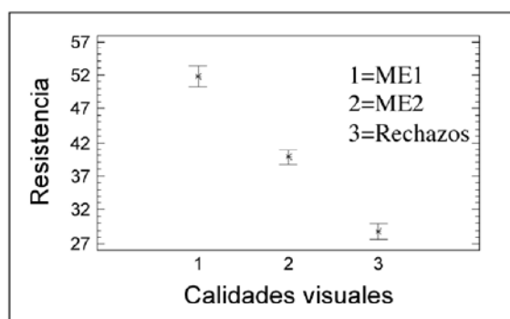
Figura 2. Análisis ANOVA calidad visual-resistencia a la flexión ( \text{N/mm}^2 )
