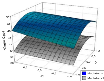
Figura 4: Variación del número Kappa según el tiempo de operación y la concentración de lacasa en dos niveles de concentración del mediador (siringaldehído).
