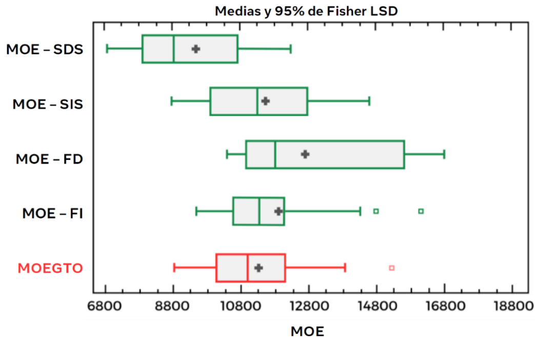
Figura 6: Comparación de los valores del MOE (MPa) obtenidos con cada tipo de medición (en verde) y del valor de referencia en máquina MOEGTO (MPa) (en rojo).
