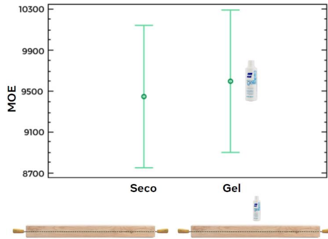
Figura 7: Comparación de las medias del MOE (MPa) obtenidas con mediciones directas en seco (MOESDS) y con gel (MOESDG), mostrando el efecto del gel de acoplamiento (Sylvatest).
