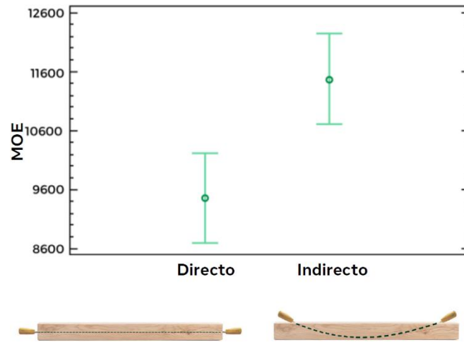
Figura 9: Comparación de las medias del MOE (MPa) obtenidas con mediciones directas (MOESDS) y mediciones indirectas (MOESIS) en seco, mostrando el efecto de la disposición de los palpadores (Sylvatest).
