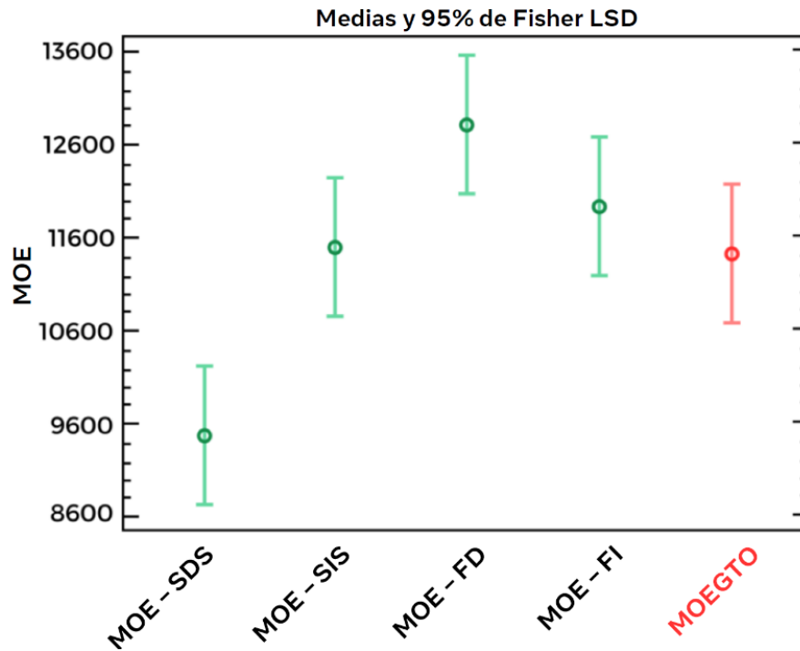
Figura 13: Comparación de las medias del MOE (MPa) obtenidas con los distintos tipos de mediciones y del valor de referencia en máquina (MOEGTO), resaltado en rojo.
