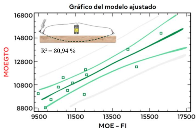
Figura 15: Gráfico del Modelo Ajustado entre MOEGTO (MPa) y MOEFI (MPa).
