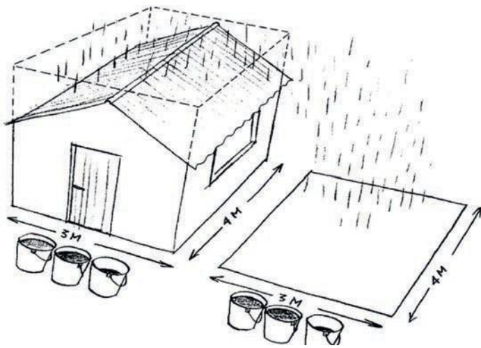
Figura 10. Gráfico de área de captación en techos con pendiente. Fuente: Worm y Hattum (2006: 29).
