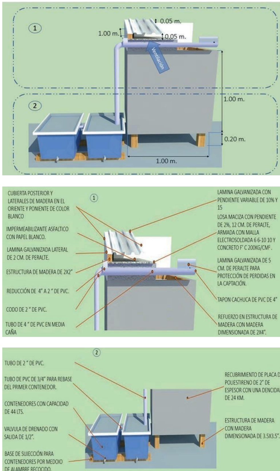
Figura 7. Gráfico del modelo TE15 (ubicación oriente). Fuente: Tobías (2019: 55).
