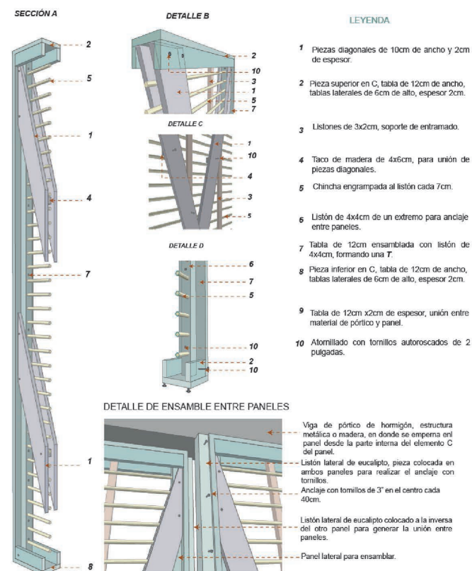
SECCIÓN Y DETALLES CONSTRUCTIVOS
