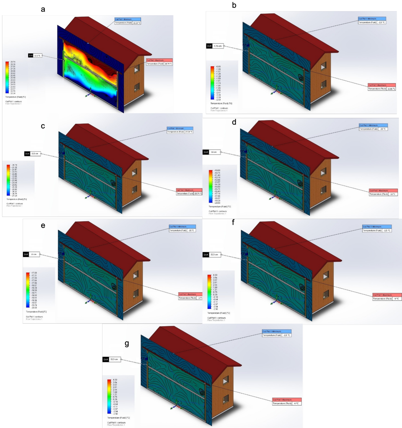
Figura 4. Comparativo de las simulaciones CFD de la casa ecológica, de acuerdo al diseño de optimización experimental donde se observa el espesor de las paredes y la escala de temperatura exterior e interior. Parte 2. Fuente: Elaboración de los autores.
