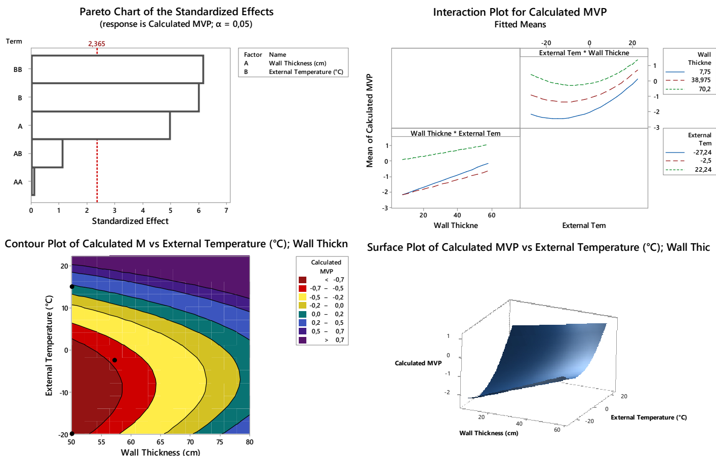
Figure 5. a) Diagrama de Pareto que identifica los efectos estandarizados. b) interacción de medias de PMV. c) gráfico de contorno que muestra los espacios de confort y desconfort térmico. d) Gráfico 3D del confort térmico en la casa ecológica. Fuente: Elaboración de los autores.
