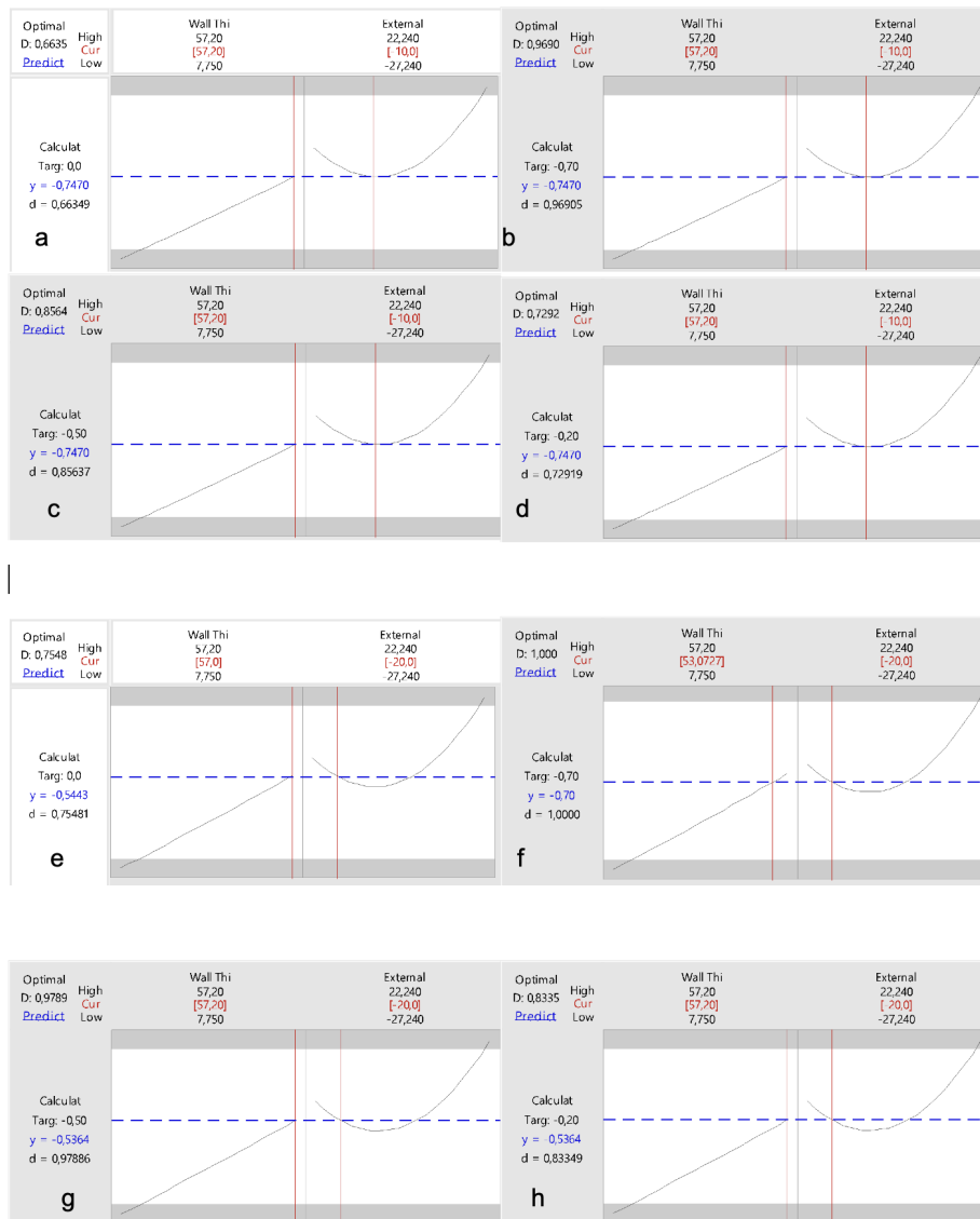
Figura 6. Optimización de grosor de pared a temperaturas ambientales extremas a -20 °C y -10 °C bajo predicción y deseabilidad aceptable. Fuente: Elaboración de los autores.
