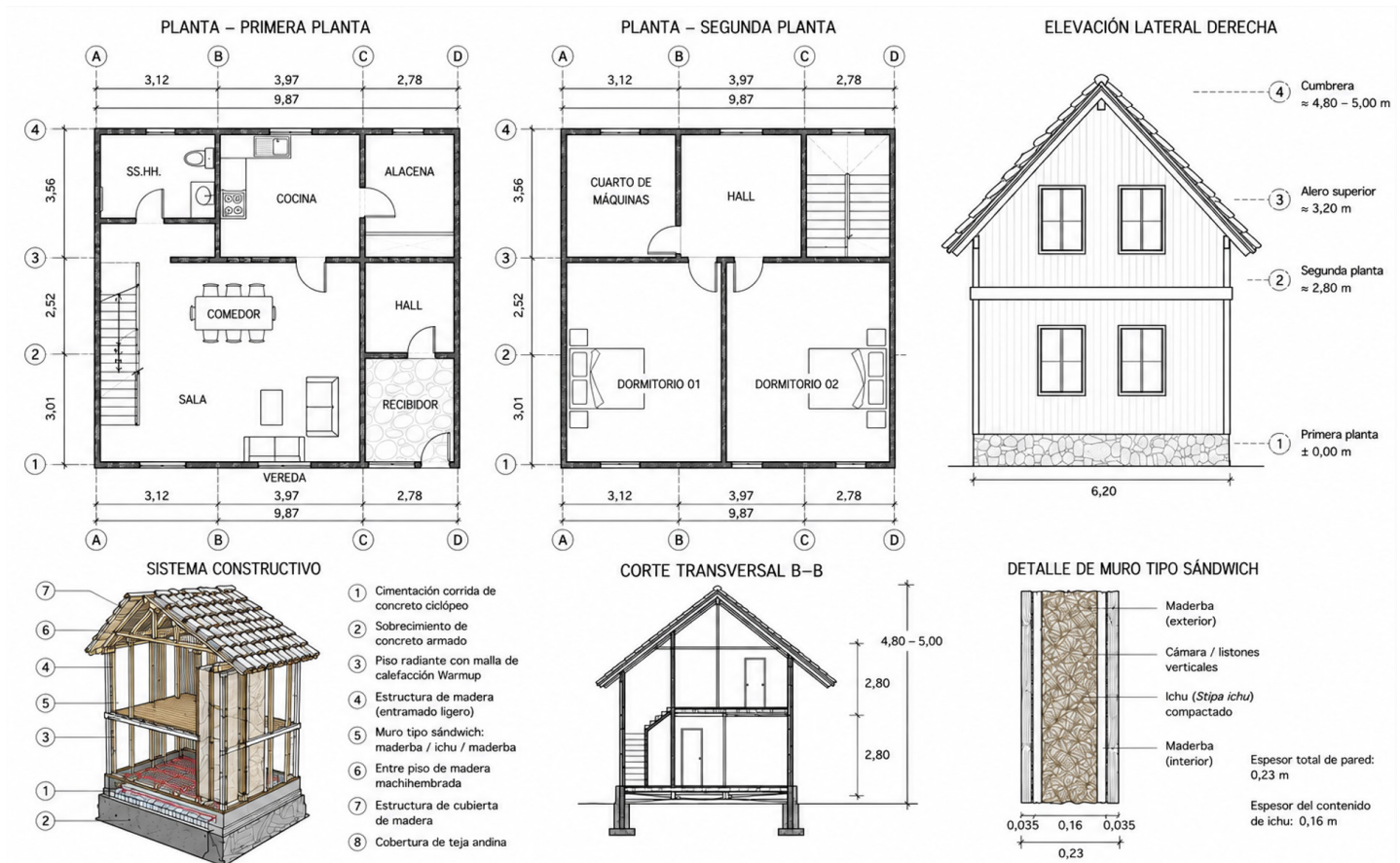
Figura 2. Esquema constructivo de la vivienda en estudio. Fuente: Elaboración por los autores.
