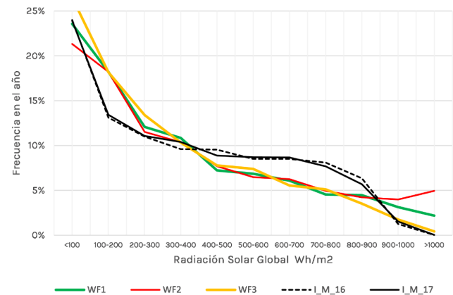
Figura 3. Comparativo de frecuencia de valores radiación solar global por rangos. Fuente: Elaboración de los autores.
