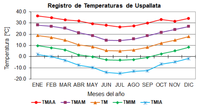
Figura 7. Temperaturas máximas y mínimas absolutas y medias mensuales para Uspallata. Fuente: Esteves Miramont (2017, p. 185).
