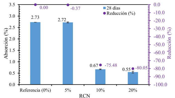
Figura 14. Absorción de las mezclas con RCN a los 28 días. Fuente: Elaboración de los autores.
