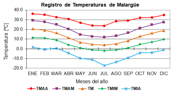
Figura 6. Temperaturas máximas y mínimas absolutas y medias mensuales para Malargüe. Fuente: Esteves Miramont (2017, p. 185).
